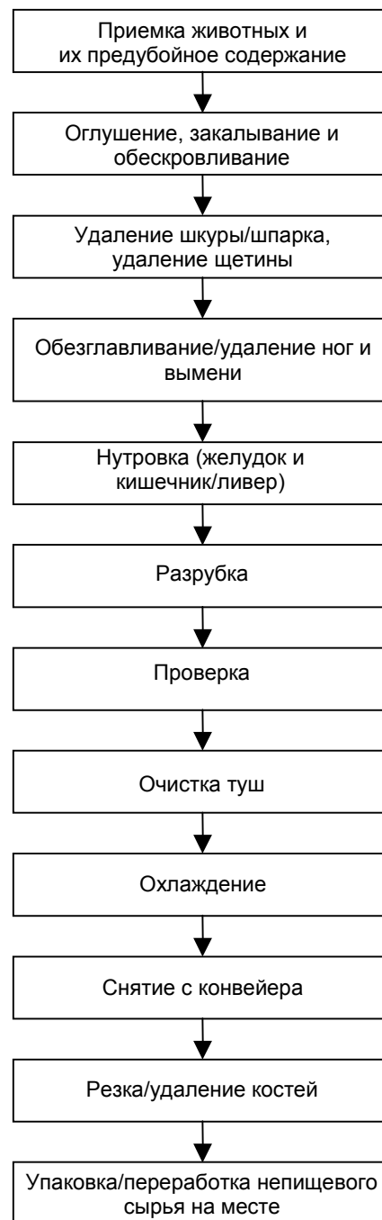
Рисунок А.1. Процесс убоя крупного рогатого скота/свиней
