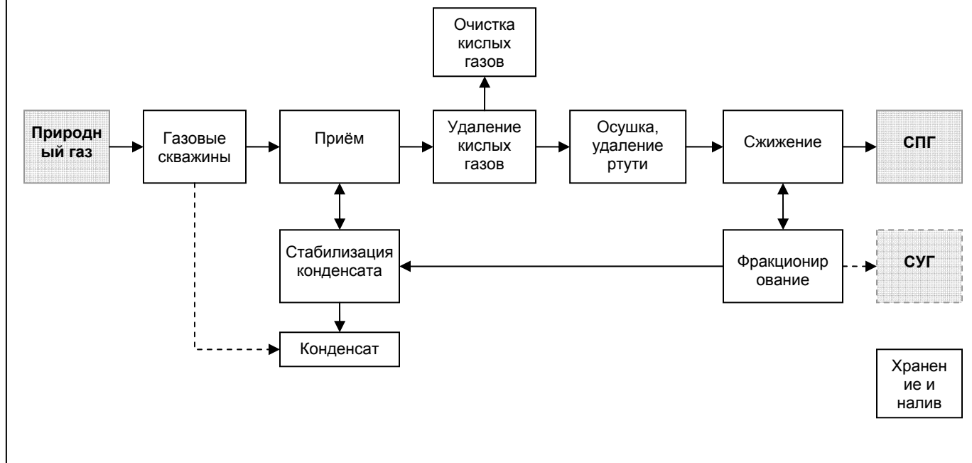
Рисунок А.1: Производство сжиженного природного газа
